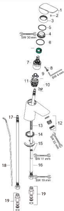
製品分解図
