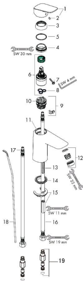
製品分解図
