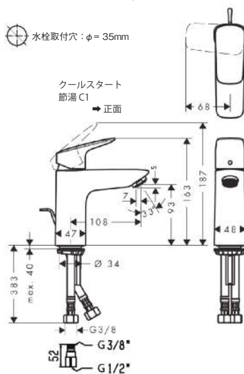
完成図
