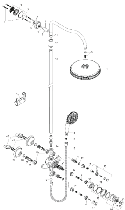
製品分解図
