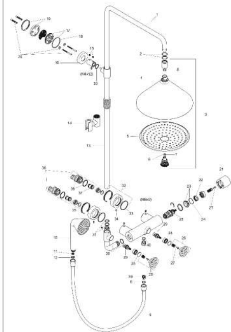
部品リスト
