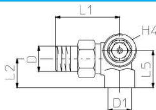
Winkelckgehäuse
