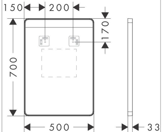
Maßzeichnung
